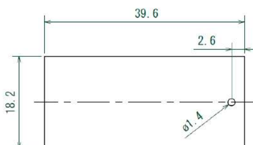
基板外形
